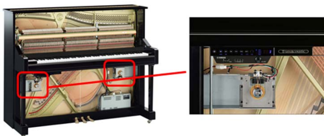
トランスデューサー(加振器)
